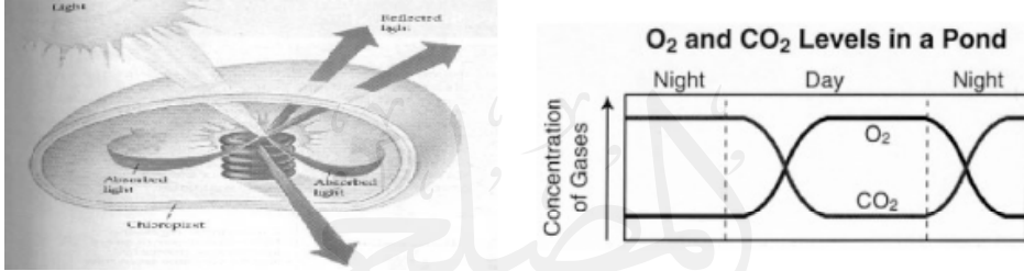
شكل (٤) : مستويات ثاني أكسيد الكربون والأوكسجين أثناء الليل والنهار في الأماكن الخضراء بالنبات
